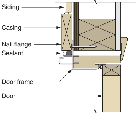
JAMB
