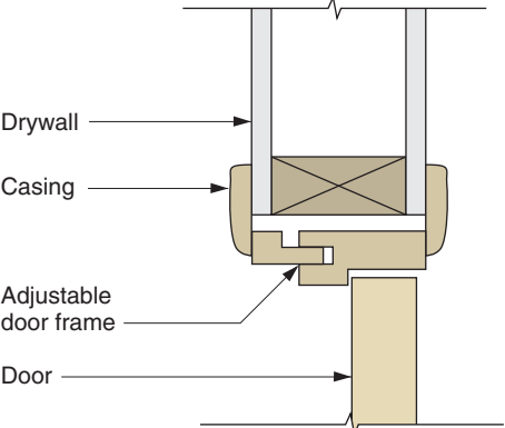
JAMB
