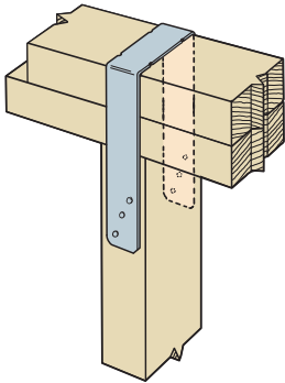
SP4 Stud Plate Tie
